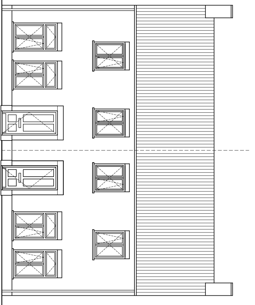
Kavel 1 voorgevel
