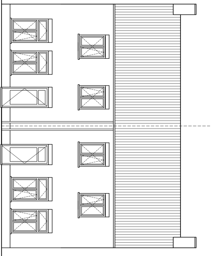
Kavel 4 achtergevel
