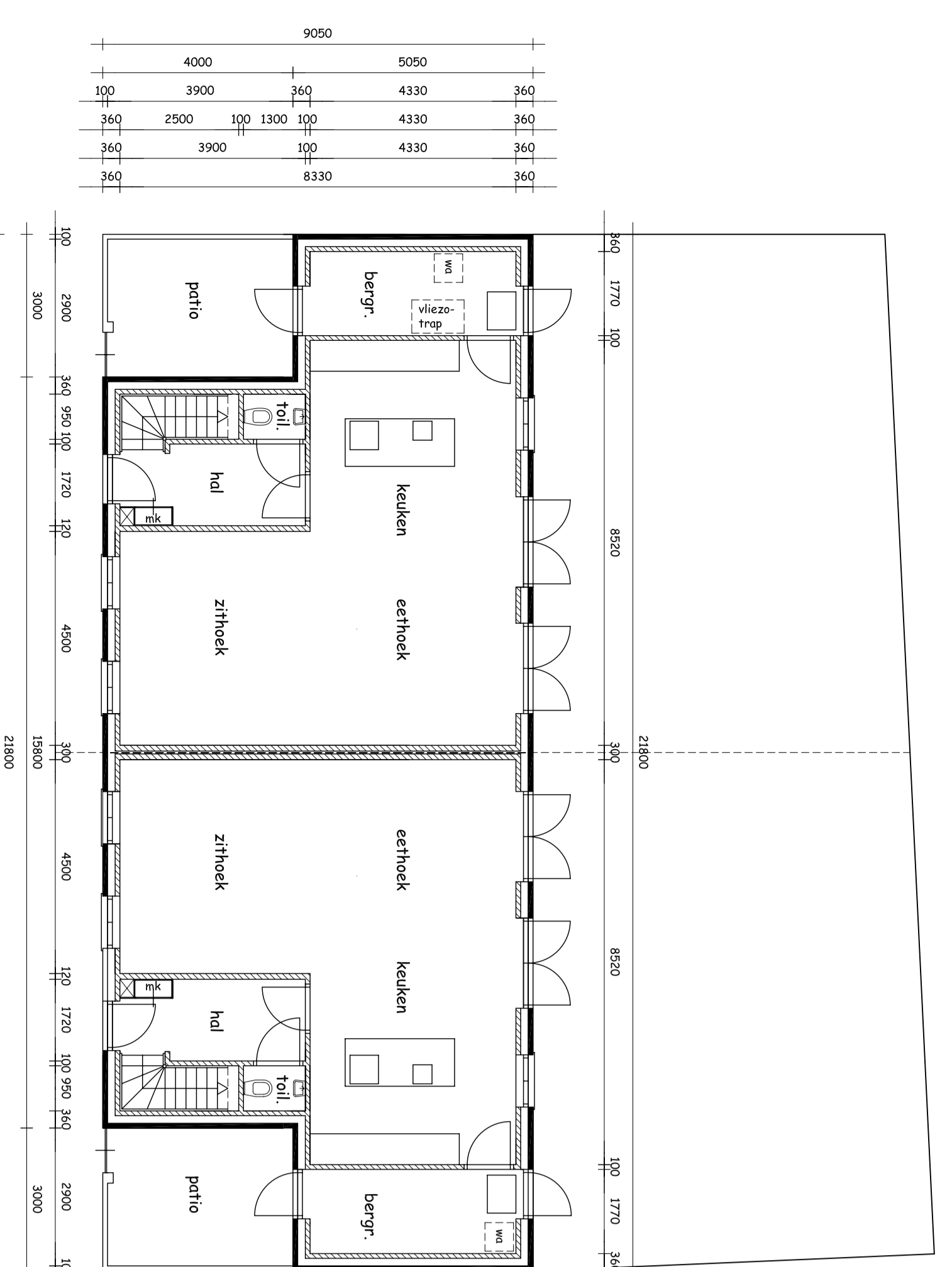
beganegrond
