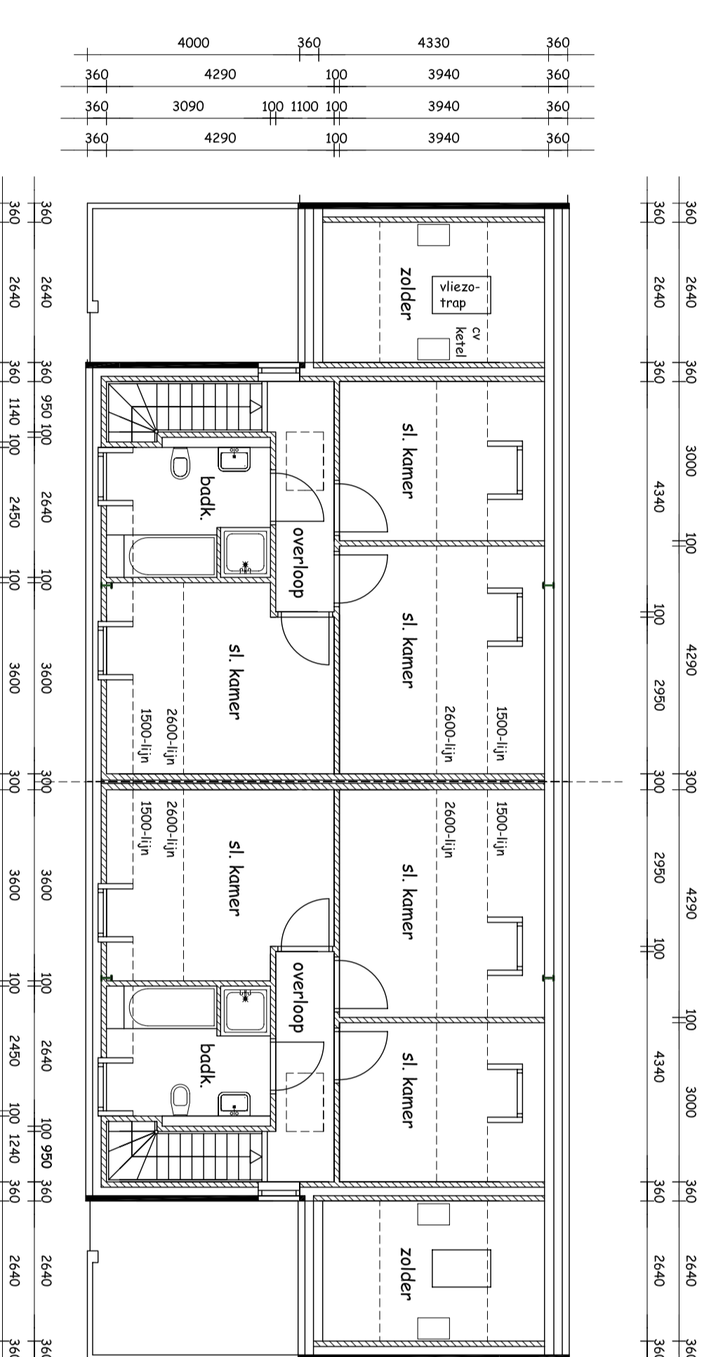
verdieping
